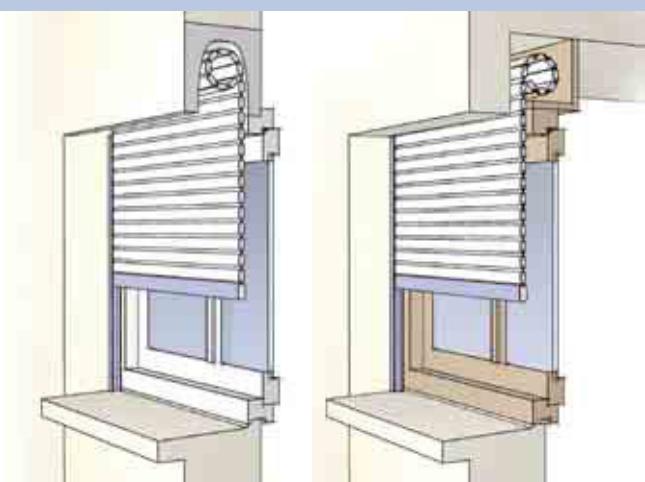
Avec coffre tunnel intégré dans la maçonnerie
