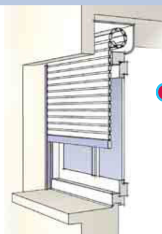
Avec coffre PVC à l'intérieur de la pièce, intégré au bloc fenêtre
