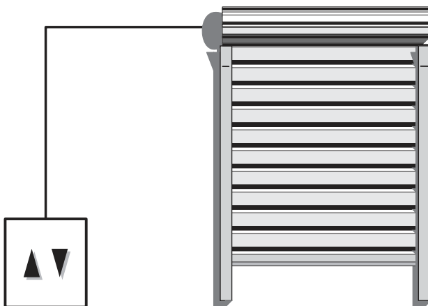
Commande individuelle : un interrupteur par volet.
