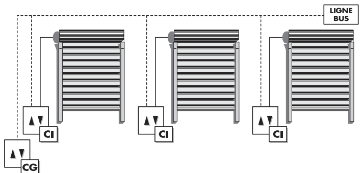
Commande individuelle et commande générale.
